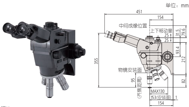
照片: FS70Z-TH (目镜、物镜、转塔为选件)
